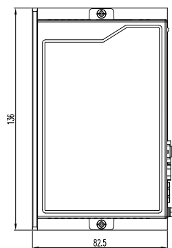
正面安装图
